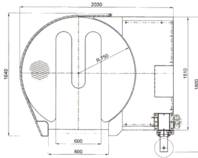
Schema utilaj FP ECO-T
