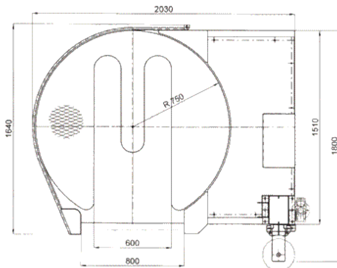
Schema utilaj FP10-T
