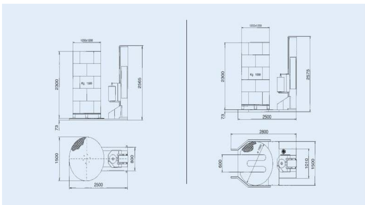
Schema utilaj
